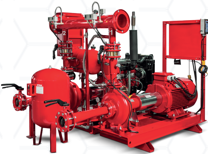
TS EN 12845 ST. FIRE PUMP
